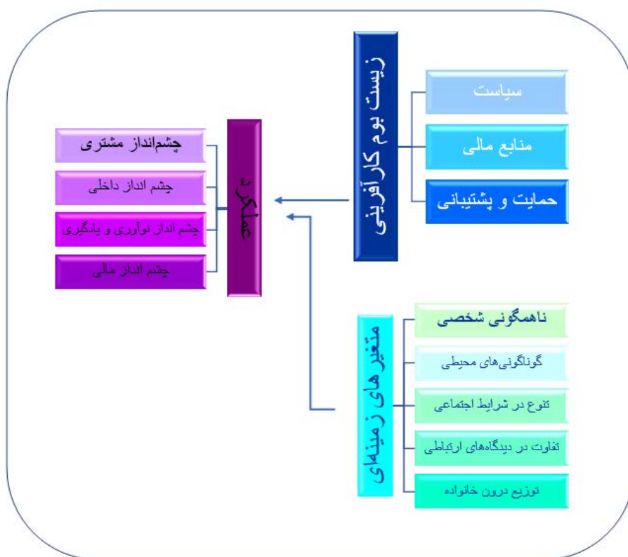
شکل ۱. چارچوب نظری
