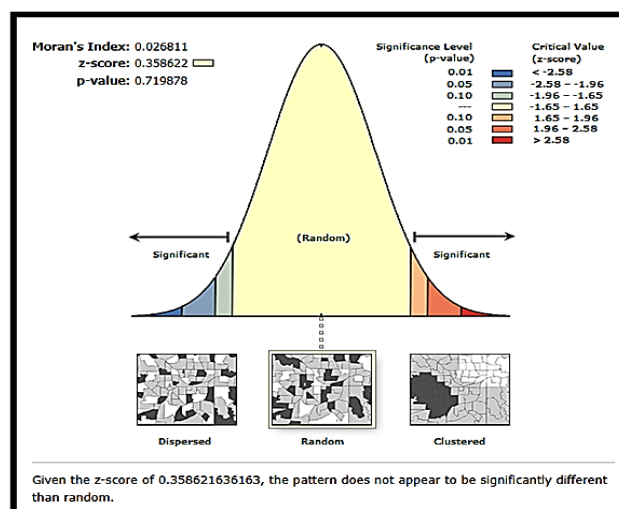
شکل ۷. مدل موران
